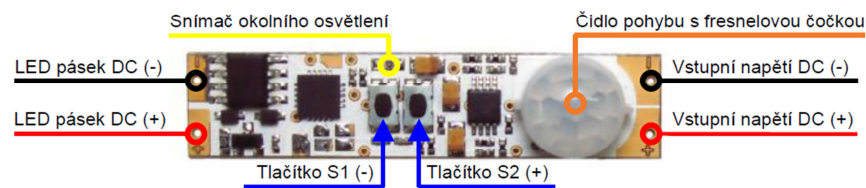
Obr.1 - Zapojení vývodů a umístění ovládacích prvků
